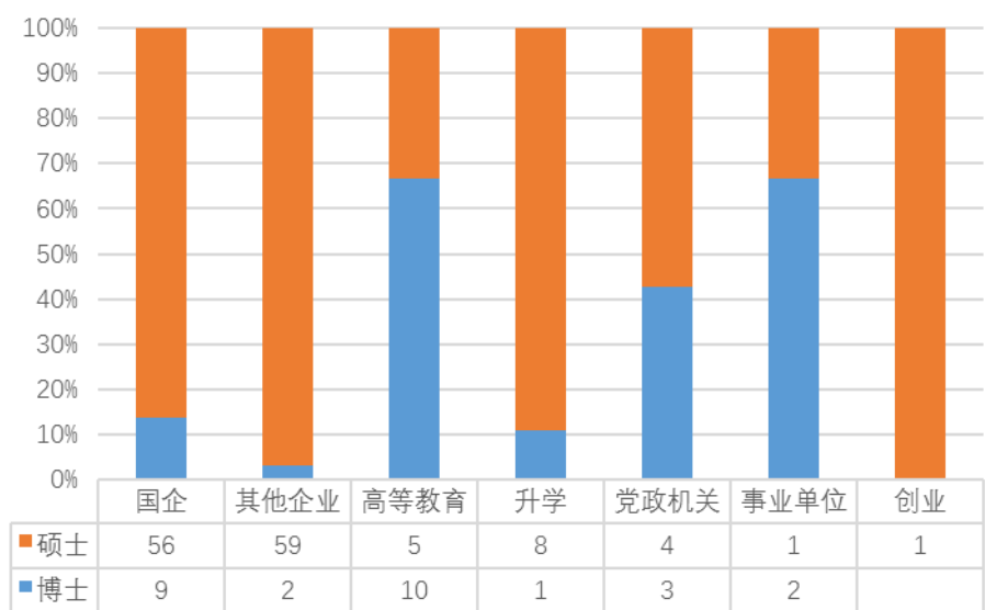
图 9 行业硕博比
